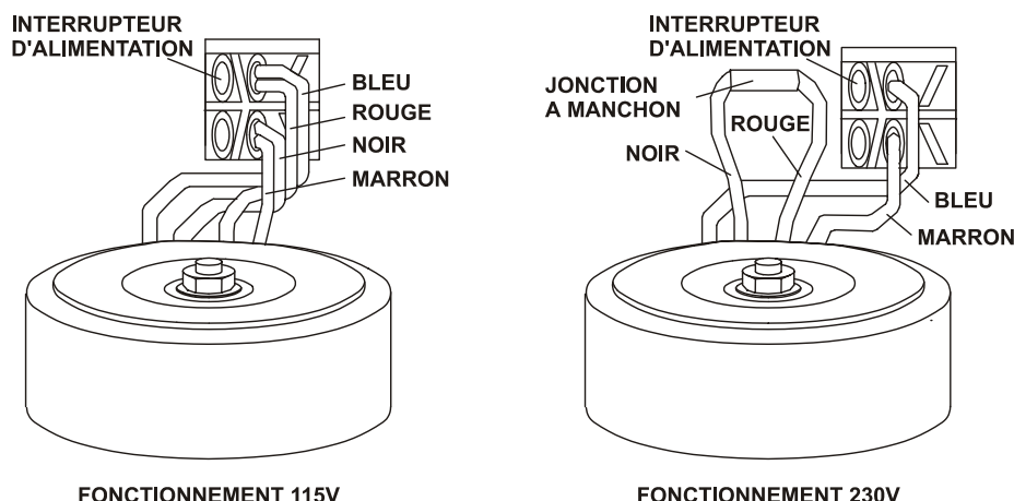
FONCTIONNEMENT 115V
