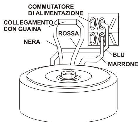
FUNZIONAMENTO 230V
