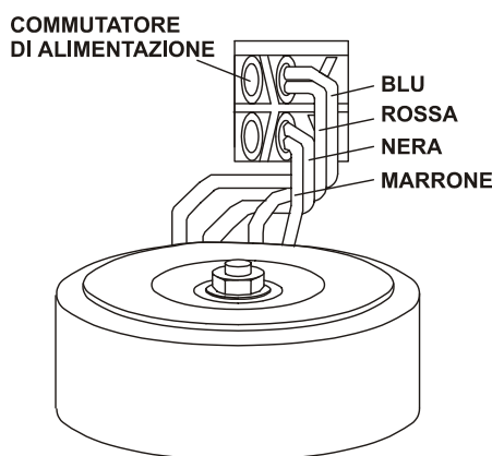
FUNZIONAMENTO 115V
